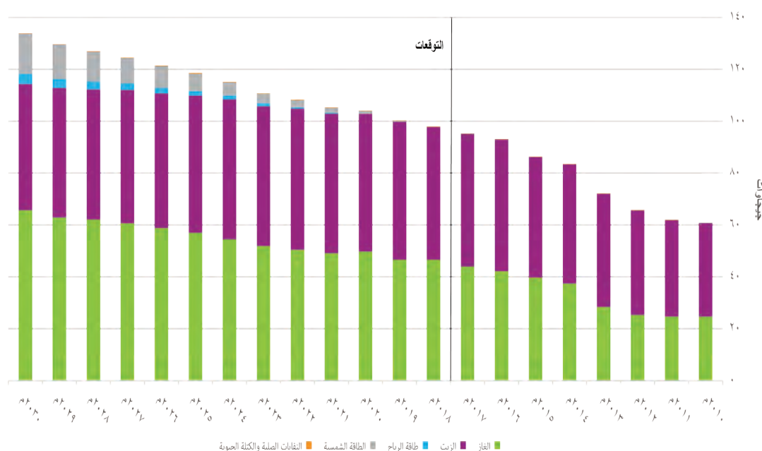
الشكل ١٢: الزيادة الفعلية والمتوقعة في الطاقة الاستيعابية لتوليد الكهرباء حسب نوع الوقود (بما في ذلك الغاز الطبيعي) المستخدم في المملكة خلال الفترة من عام ٢٠١٠م إلى عام ٢٠٣٠م
