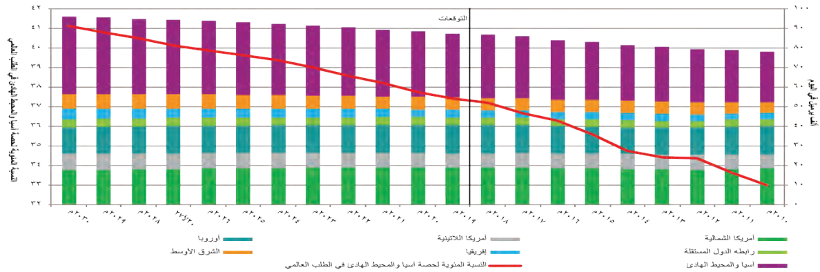
الشكل ٨: الطلب الفعلي والمتوقع على المنتجات المكررة حسب المنطقة خلال الفترة من عام ٢٠١٠م إلى ٢٠٣٠م
