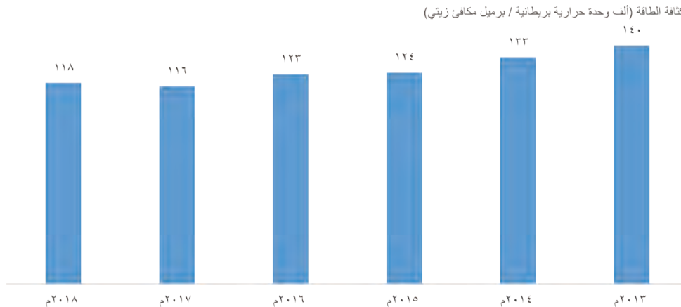
الشكل ٢٧: كثافة استهلاك الطاقة في المرافق التي تشغلها شركة أرامكو السعودية في المملكة من عام ٢٠١٣م إلى عام ٢٠١٨م
