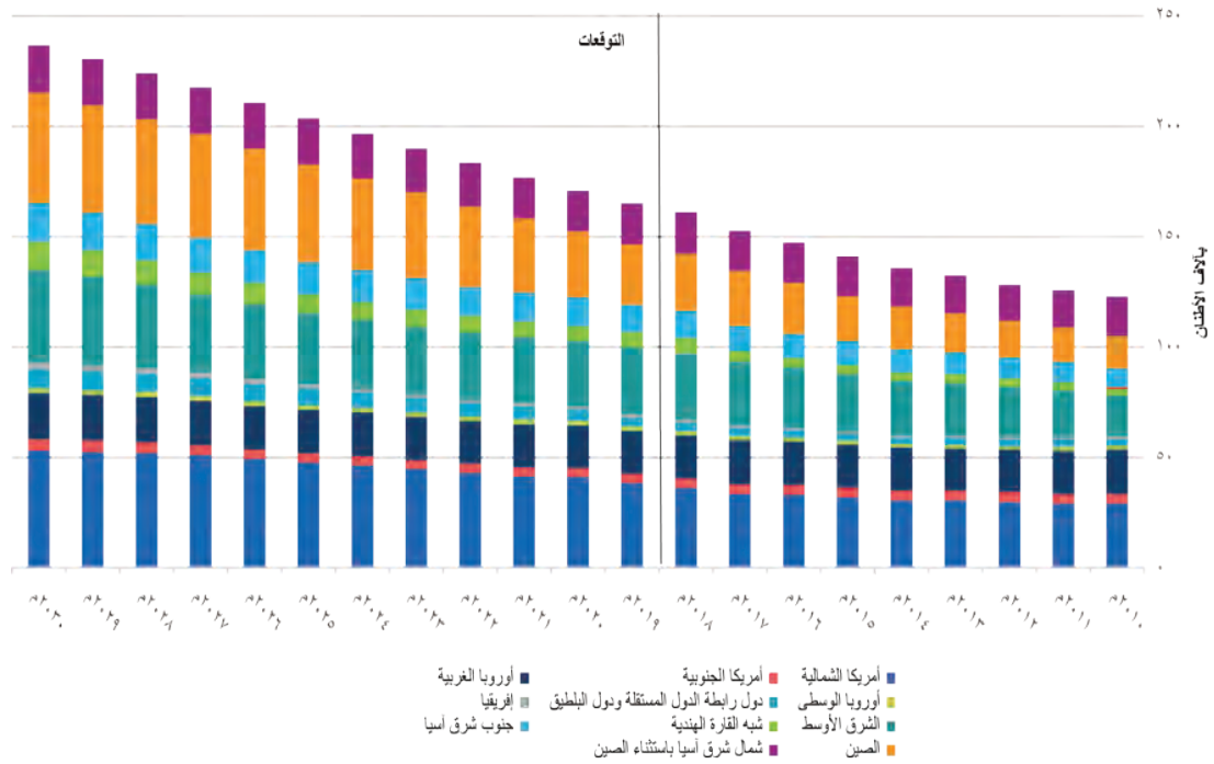
الشكل ١٠: الطلب الفعلي والمتوقع على الإثيلين عالمياً حسب المنطقة خلال الفترة من عام ٢٠١٠م إلى عام ٢٠٣٠م
