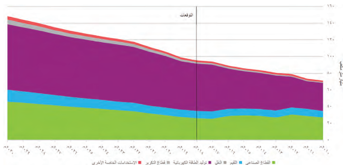
الشكل ١١: الطلب الفعلي والمتوقع على الغاز الطبيعي بالمملكة بحسب القطاع خلال الفترة من عام ٢٠١٠م إلى عام ٢٠٣٠م
